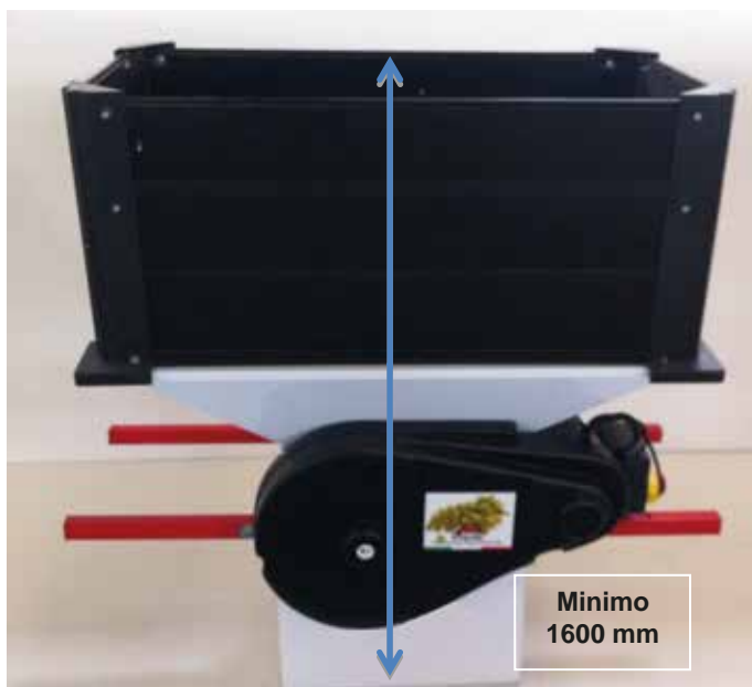
Fig. 3 Limiti dimensionali nel posizionamento
