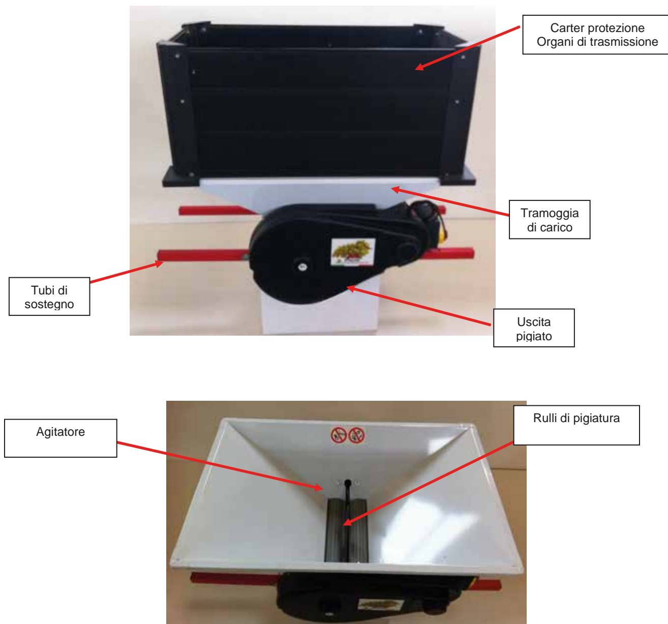
Fig. 1 Elementi fondamentali della PIGIATRICE A MOTORE
