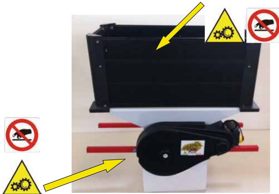
Fig. 2 Ubicazione degli organi mobili
